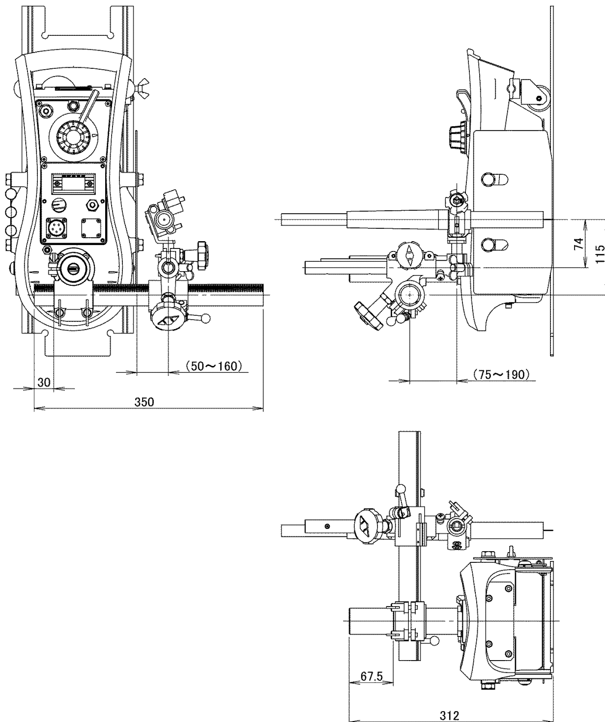
IK-12 NEXT 搭載外観図
